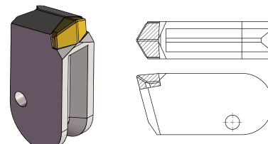
双轮铣刀 -N
