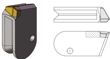
双轮铣刀 -U
