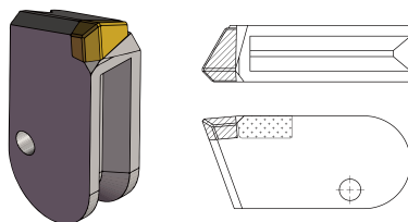
双轮铣刀 -S
